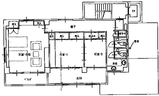
4 階図面
